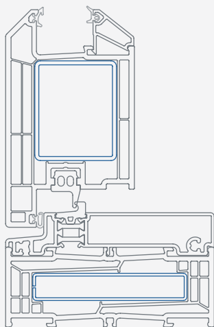
Huisdeur NL 71 Elite naar buiten draaiend
