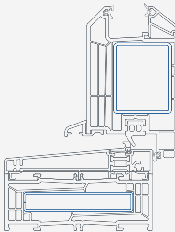
Huisdeur NL 71 Elite naar binnen draaiend
