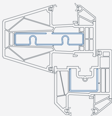
Verbinding tussen staande en liggende delen van het kozijn
