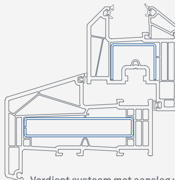
Verdiept systeem met aanslag voor montage aan stelkozijnen
